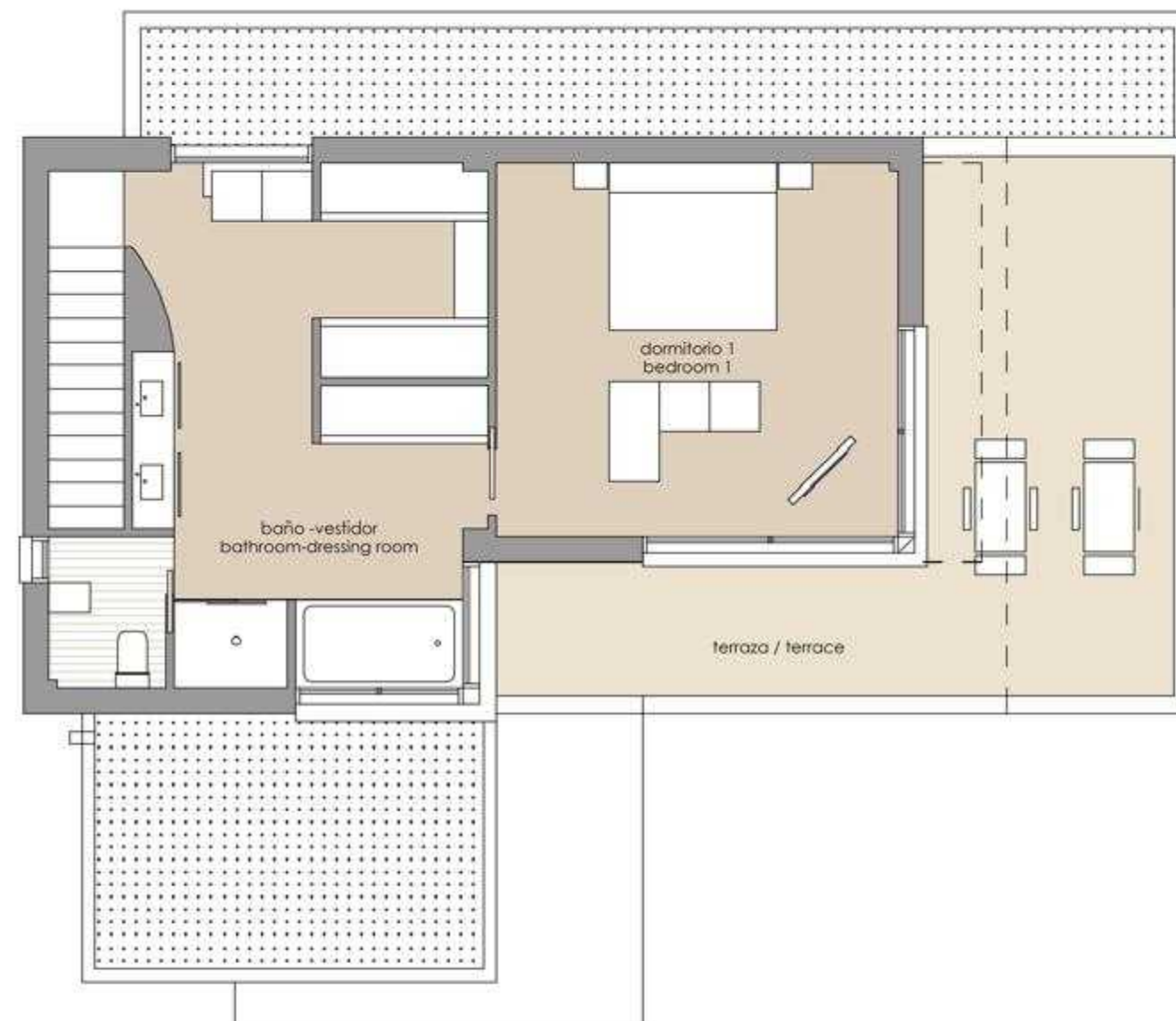
PLANTA PRIMERA | FIRST FLOOR
